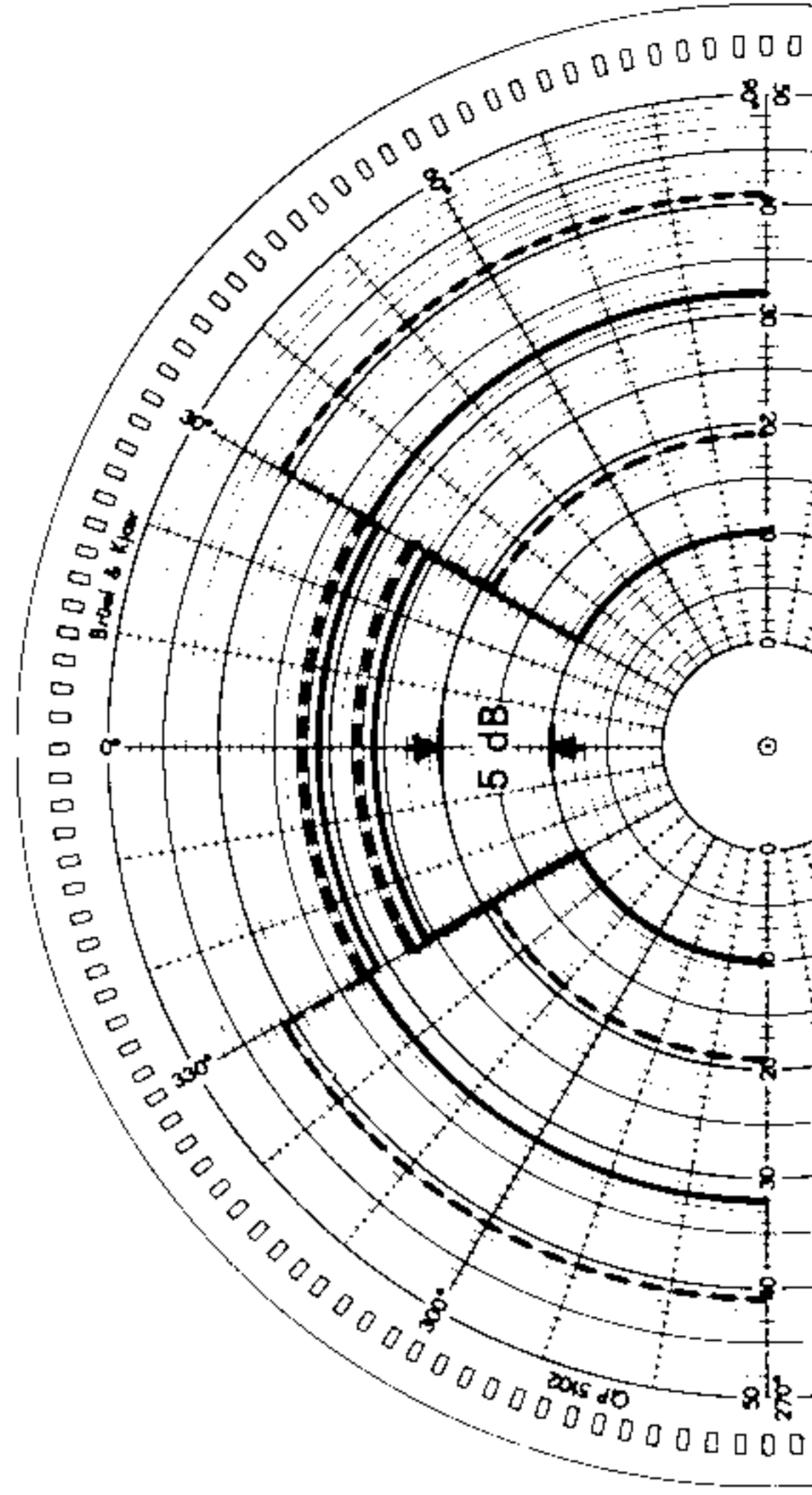
8 kHz — 12,5 kHz 760074
